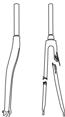
Figura 2.5: A sinistra: Quando vengono sovraccaricate le forcelle in metallo si possono deformare. A destra: Le forcelle in carbonio resistono a sollecitazioni più elevate, ma cedono completamente in caso di sovraccarichi.
