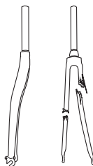
Rysunek 2.5: Po lewej: Wygięcie metalowego widelca przy przeciążeniu. Po prawej: Widelec z włókna węglowego wytrzymał znacznie większe obciążenie, ale doszło do złamania przy przeciążeniu.
