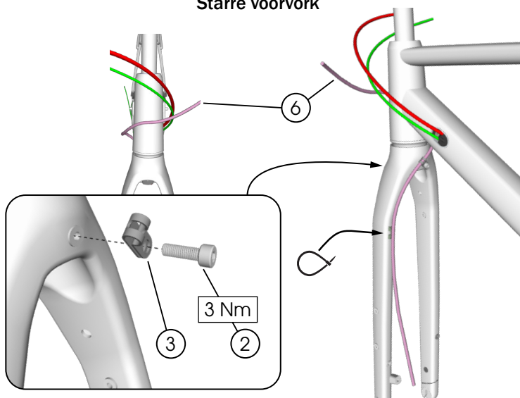
Starre voorvork
