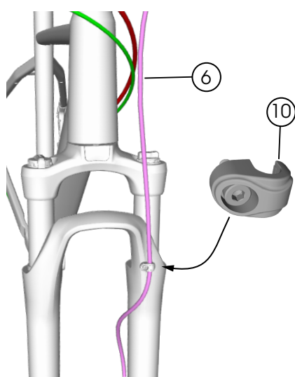
Geveerde voorvork
